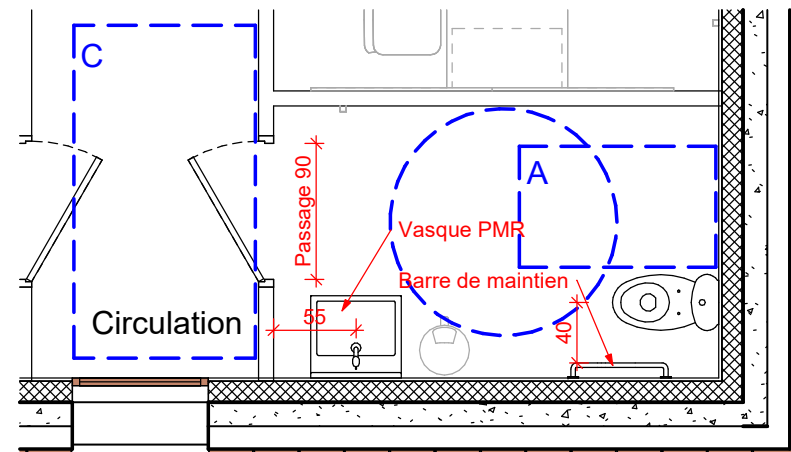
ZOOM 2: 1/50 AFA Niveau 0 Sanitaire personnel
