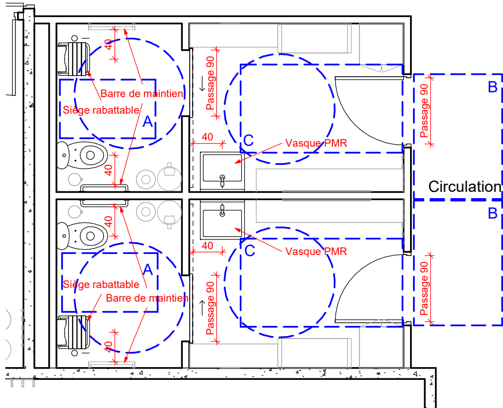
ZOOM 3: 1/50 PHE Niveau 0 Vestiaires personnel
