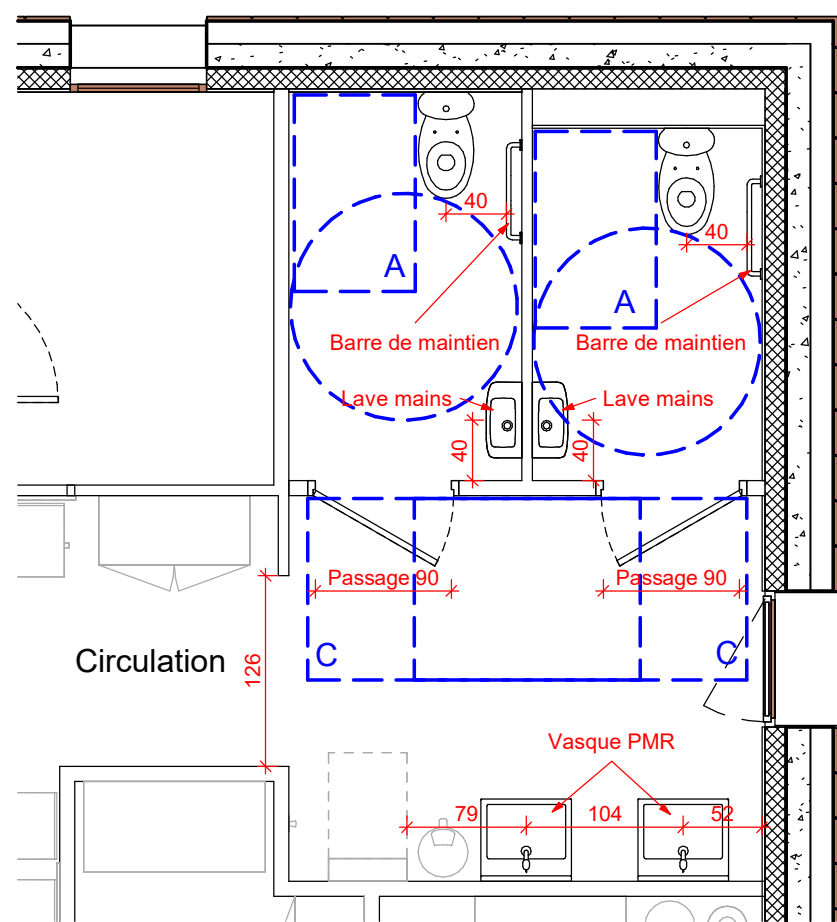
ZOOM 1: 1/50 AFA Niveau 0 Sanitaires visiteurs
