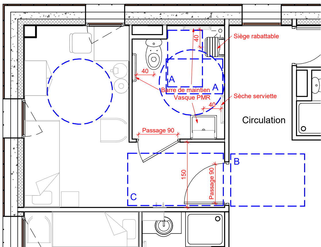
ZOOM 4: 1/50 PHE Niveau 1 Chambre individuelle PMR
