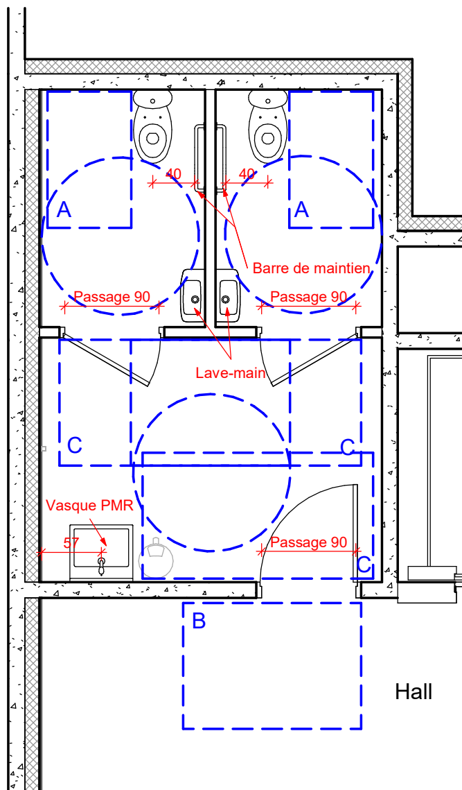
ZOOM 2: 1/50 PHE Niveau 0 Sanitaires convives
