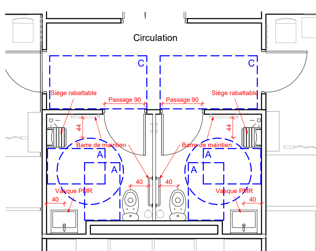
ZOOM 5: 1/50 PHE Niveau 1 Vestiaires personnel
